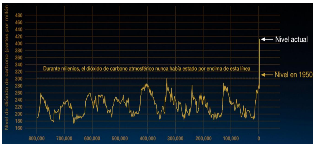
Gráfico 2. Concentraciones de CO 2 en partes por millón (ppm) desde hace 800,000 años. Fuente: NASA, 2019.
